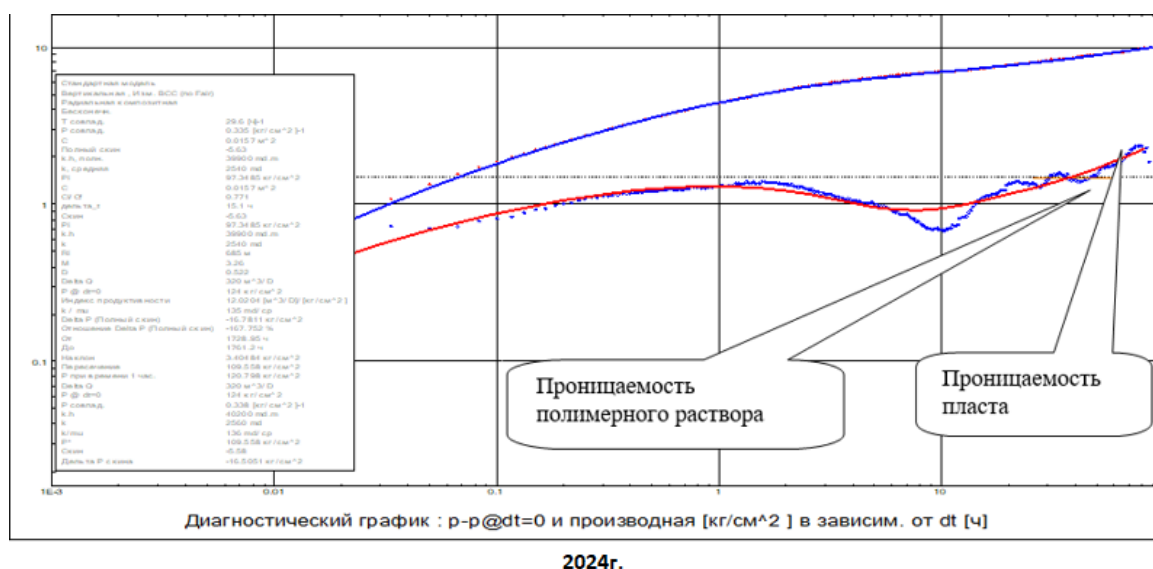
Рисунок 2 - Изменение забойного давления во времени (КПД) в логарифмических координатах и ее производная по скважине №1059 после ПЗ
