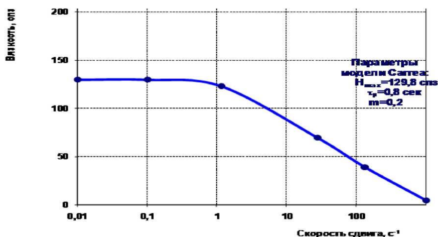
Рисунок 1 - Зависимость вязкости раствора полимера от скорости сдвига
