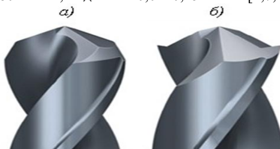
Рисунок 2 - Сверла двойной заточки (а) и (б) с острыми кромками на боковой поверхности для эмалирования полимерных композиционных материалов.
