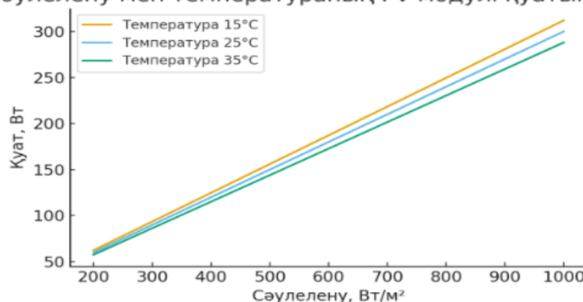
Сурет 1 — Жарықтандыру және температураның PV-модуль қуатына әсері
