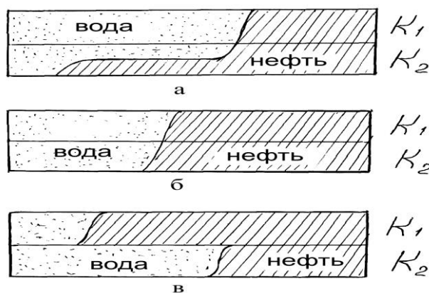
1 сурет. Екі қабатты қабаттан ығысу фронтының конфигурациясы
