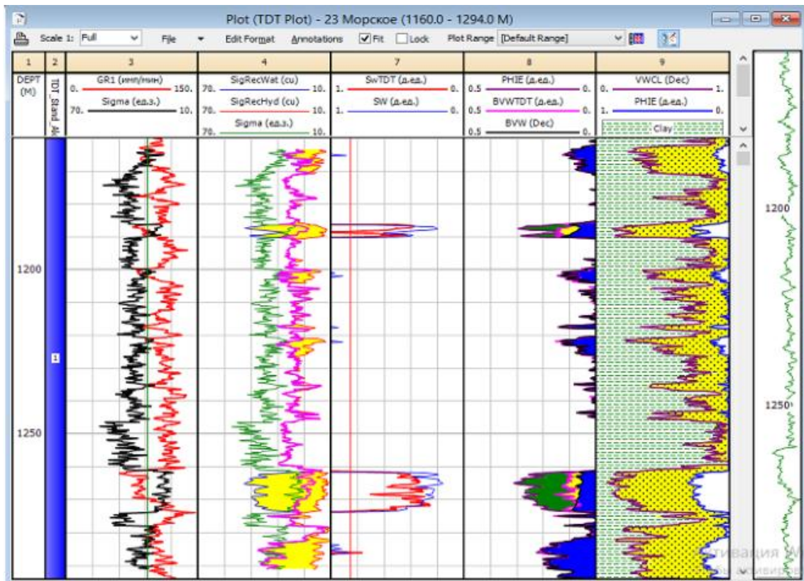
Рисунок 1 – «Interactive Petrophysics»
