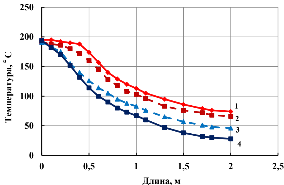
Рисунок.1. Распределение температуры по длине слоисто-неоднородного пласта после закачки горячей воды 1,4 —высоко- и малопроницаемые изолированные слои, соответственно (опыт №3). 2,3 - высоко- и малопроницаемые сообщающиеся слои, соответственно (опыт №4)
