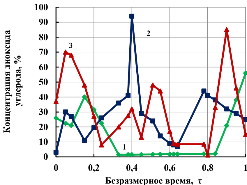
Рисунок 4. Изменение концентрации \text{CO}_2 образованный в предварительно нагретом пласте до 200^\circ\text{C} при закачке раствора карбамида 1,2,3 – 1; 7; 10% раствор карбамида
