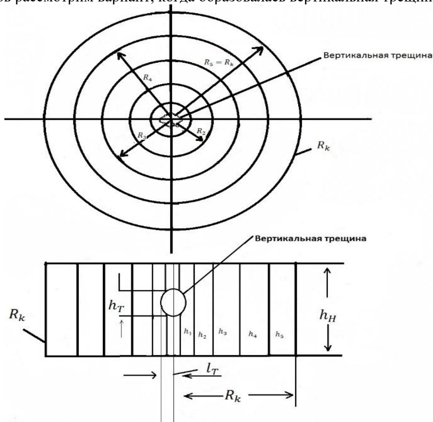
Рисунок 2. Схема расположена вертикальной трещины в зонально неоднородном пласте
