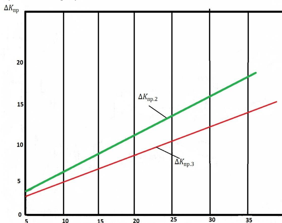
Рисунок 3. Зависимость изменения \Delta K_{\text{пр}} от соотношения \frac{K_{1\text{тр}}h_{\text{тр}}}{K_1h_n}
