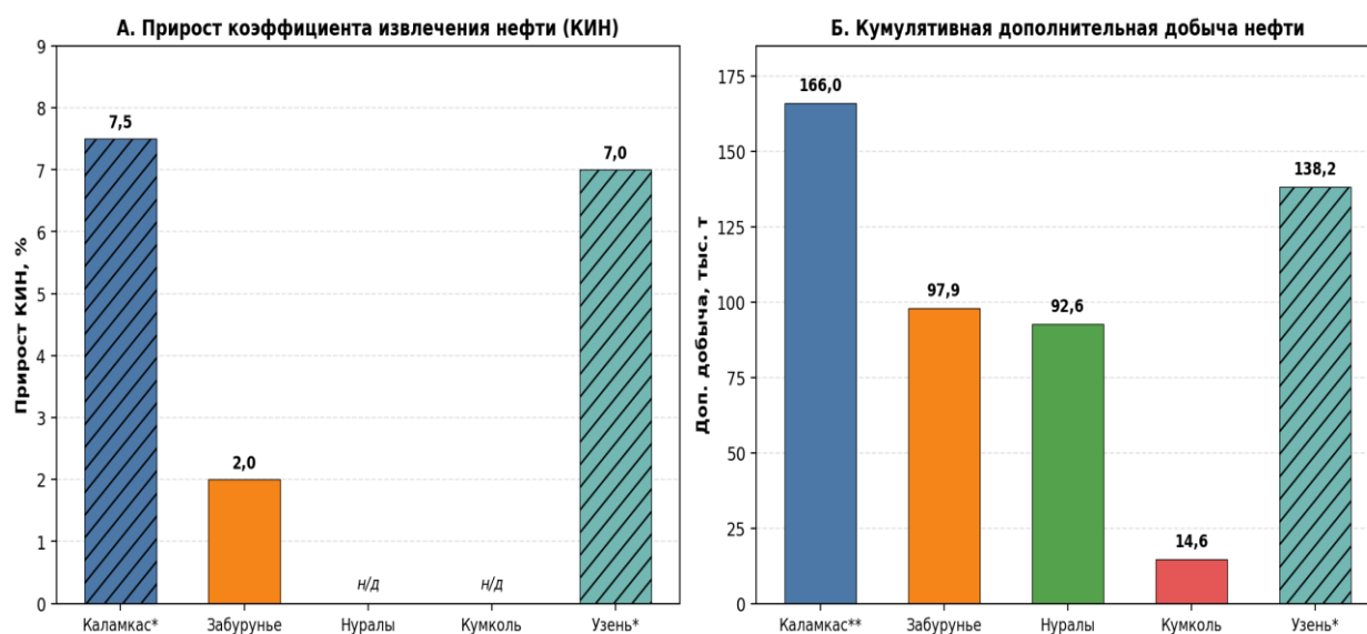
Рисунок 2 – Результаты применения полимерного заводнения на месторождениях Казахстана: А – фактический и прогнозный прирост КИН; Б – кумулятивная дополнительная добыча нефти
