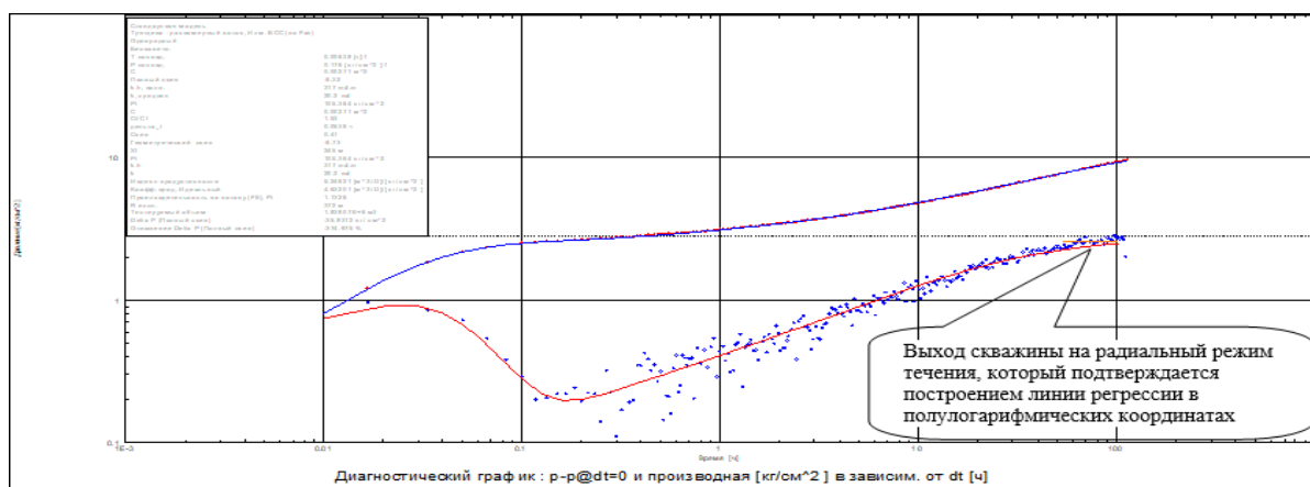
Рисунок 1 – Изменение забойного давления во времени (КПД) в логарифмических координатах и ее производная по скважине №1059 до ПЗ
