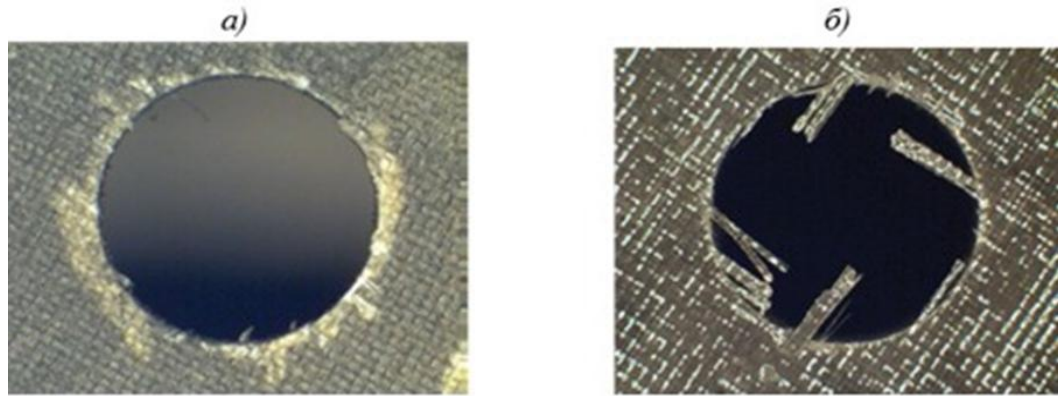
Рисунок 1 - Локальное отслаивание слоев материала (а) и срезание волокон на внутренней поверхности отверстия из-за нарушения режимов резания при сверлении (б) при неправильной осевой подаче инструмента при сверлении.
